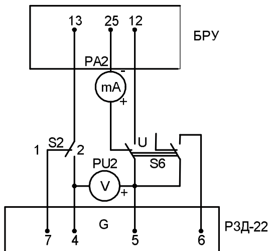
Рисунок К.2 – для исполнений -06...-09
