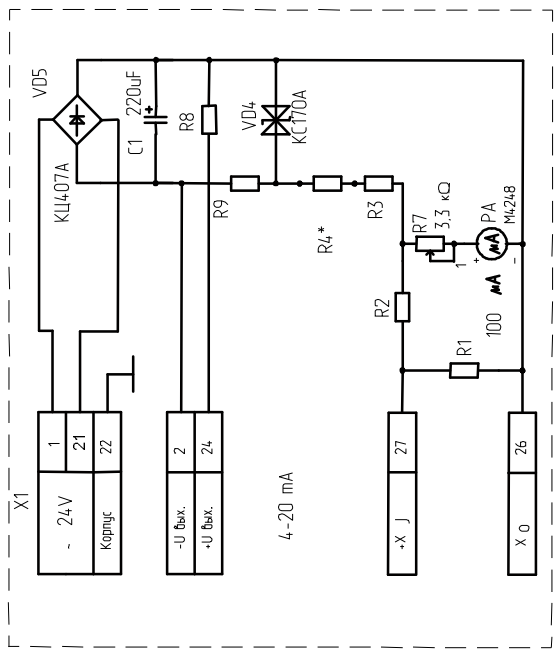
Приложение Д (обязательное) Схема электрическая принципиальная БРУ-32 (для исполнений -00...-05)
