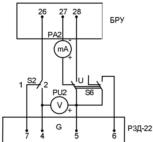
Рисунок К.1 – для исполнений -00...-05
